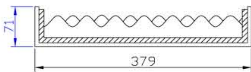
B-B
