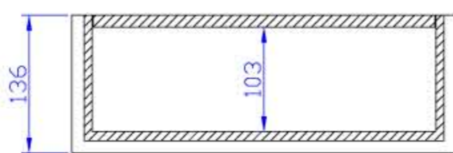
B-B
