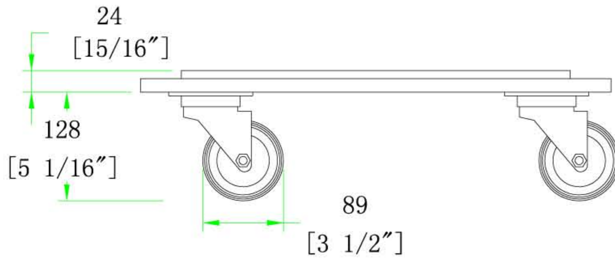
A-A VIEW
