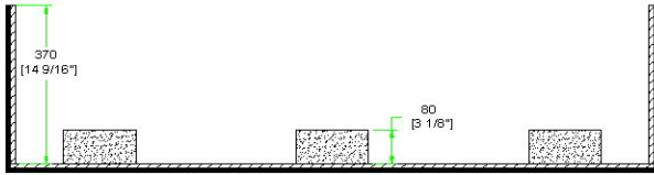
A-A VIEW
